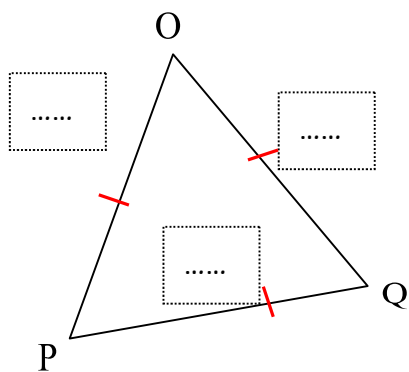
Triangle équilatéral
