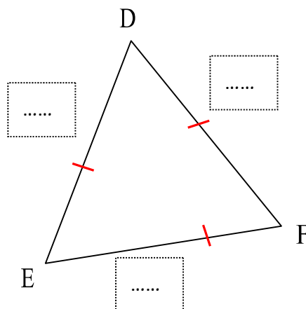
Triangle équilatéral
