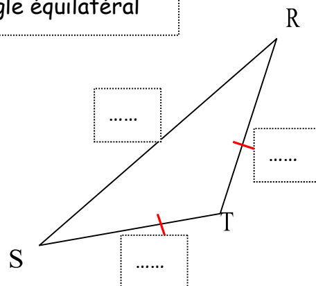
Triangle isocèle
