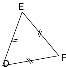
Équilatéral
