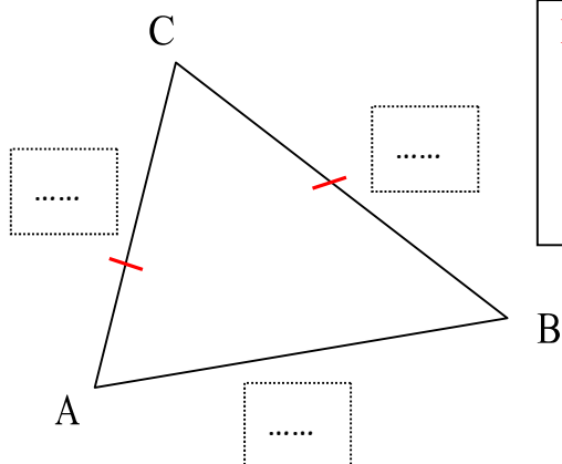
Triangle isocèle
